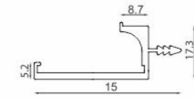
AVAP 1069 Aluminium Edge Golla Profile Size : 3000mm
