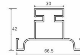
AVAP 1094 Aluminium Edge Golla Profile Size : 3000mm
