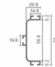
AVAP 116 Aluminium Edge Golla Profile Size : 3000mm
