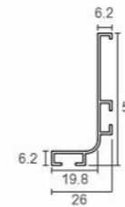
AVAP 115 Aluminium Edge Golla Profile Size : 3000mm
